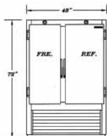
ELEVATION
